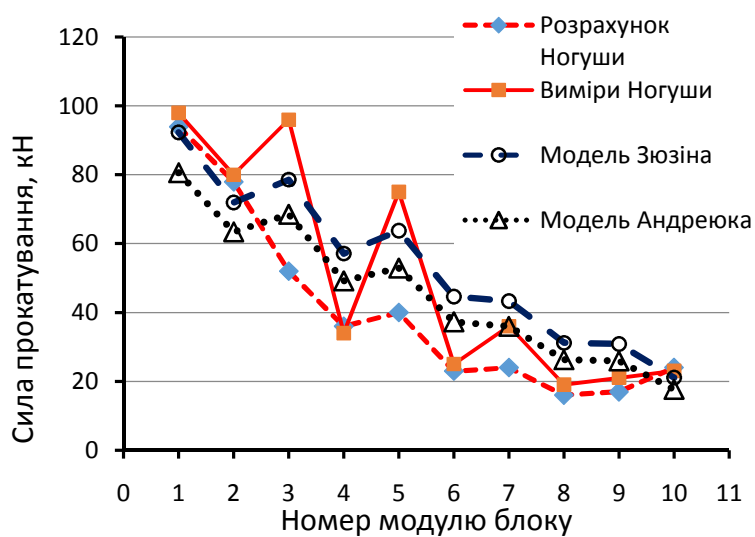
Рис. 1. Порівняння експериментальних та розрахованих значень сили прокатування в десяти модульному блоці 200
