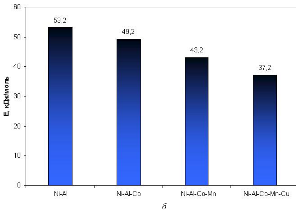
Рис. 1. Дослідження кінетики окислення оксиду вуглецю: а — залежність ефективного коефіцієнта швидкості реакції окислення оксиду вуглецю від температури; б — значення енергії активації
