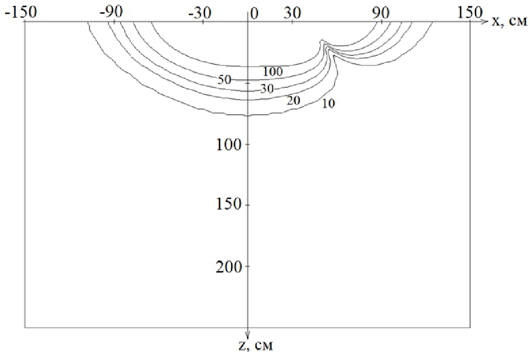
Рис. 2. Розподіл абсолютної величини щільності електромагнітних сил ( \text{H/m}^3 ) у ванні трьохелектродної УКП змінного струму
