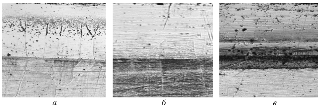
Рис. 3. Мікроструктури легованих алітованих покриттів в залежності від виду легування, на технічному залізі отриманих при t_{\text{п}} = 1000 °С, \tau_{\text{в}} = 60 хв.: а — Cr ( \times 100 ); б — Ti ( \times 100 ); в — Si ( \times 100 ).
